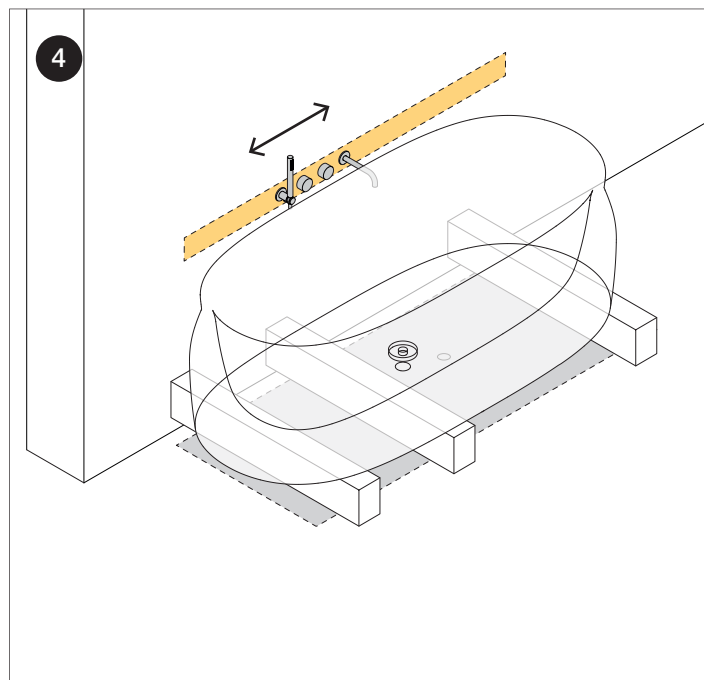
POZZETTO NORMALE / NORMAL CAVITY
