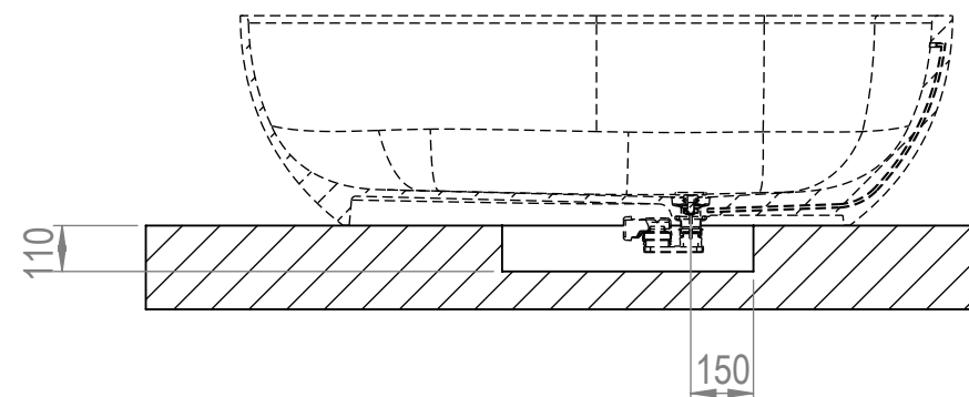
DIMENSIONI FORO POZZETTO FLOOR RECESS SIZE
