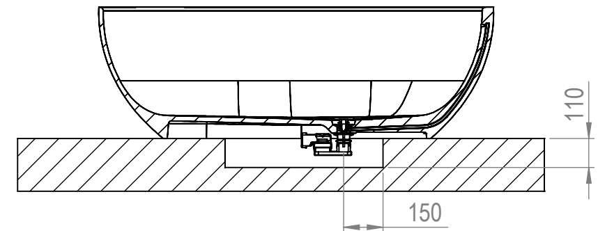
DIMENSIONI FORO POZZETTO FLOOR RECESS SIZE
