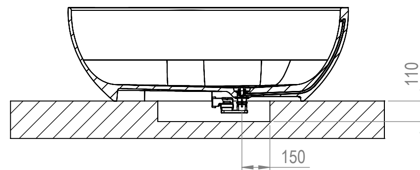
DIMENSIONI FORO POZZETTO FLOOR RECESS SIZE
