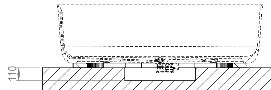
DIMENSIONI FORO POZZETTO FLOOR RECESS SIZE
