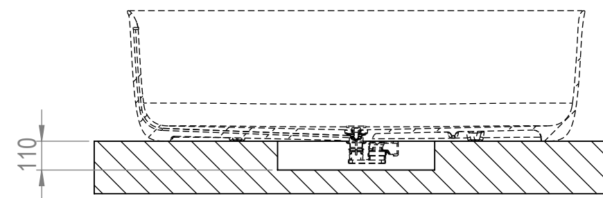
DIMENSIONI FORO POZZETTO FLOOR RECESS SIZE
