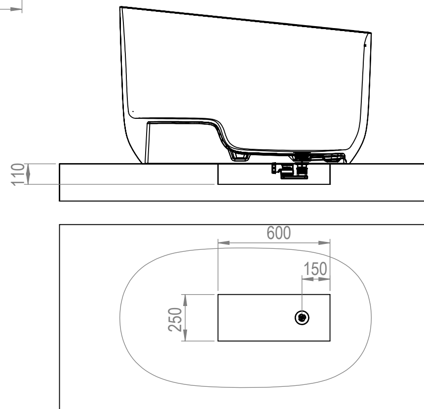
DIMENSIONI FORO POZZETTO FLOOR RECESS SIZE
