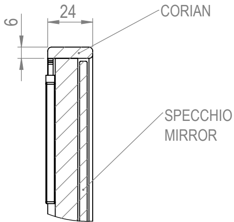
DETTAGLIO F SCALA 1 : 2
