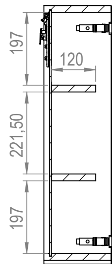
SEZIONE F-F
