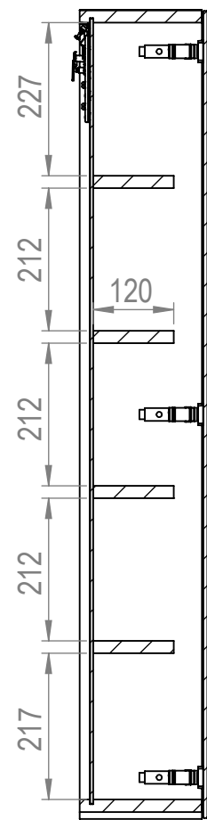
SEZIONE E-E
