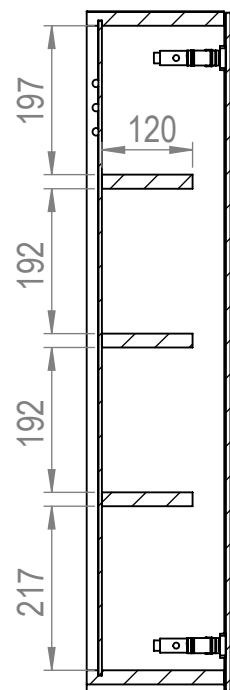
SEZIONE D-D
