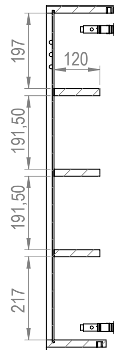
SEZIONE A-A
