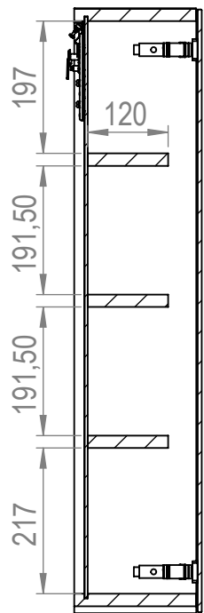
SEZIONE C-C
