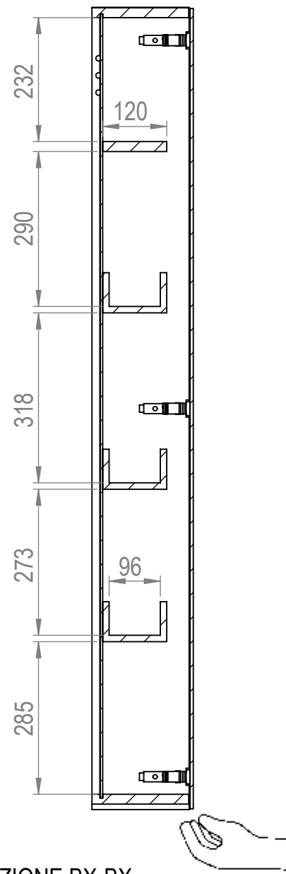
SEZIONE BX-BX
