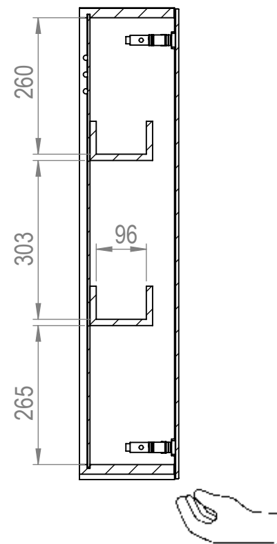
SEZIONE BO-BO
