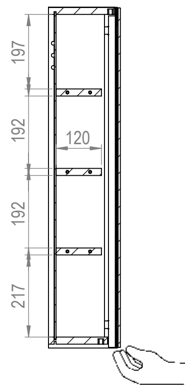
SEZIONE BY-BY
