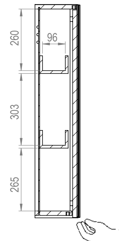
SEZIONE BZ-BZ
