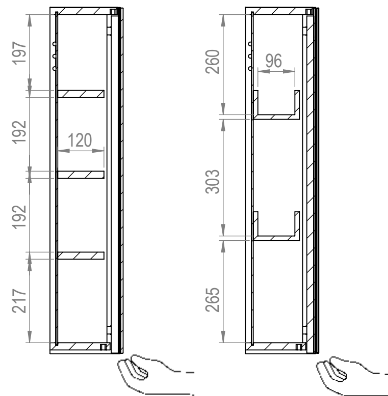
SEZIONE BM-BM
