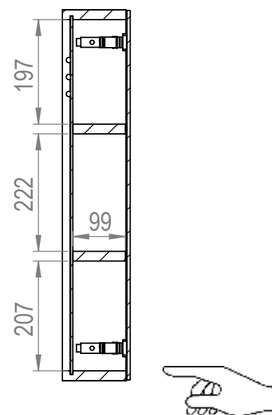
SEZIONE I-I
