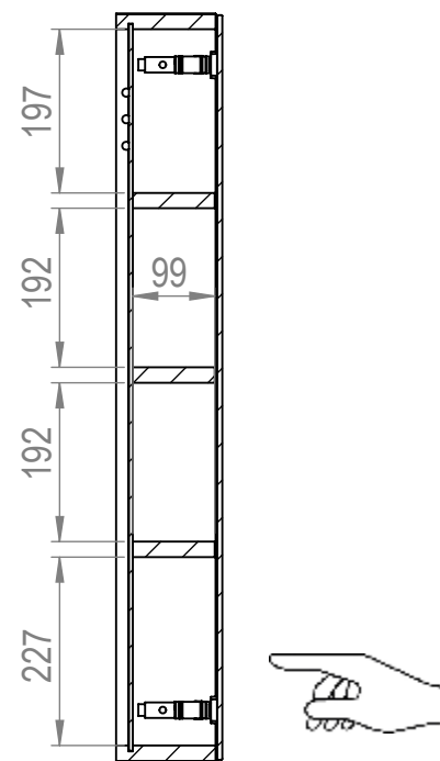
SEZIONE E-E
