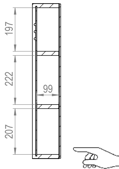
SEZIONE A-A
