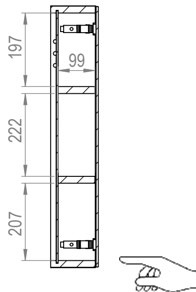
SEZIONE B-B
