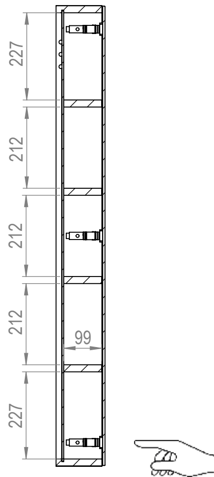
SEZIONE H-H
