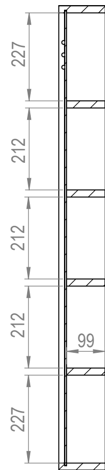
SEZIONE G-G
