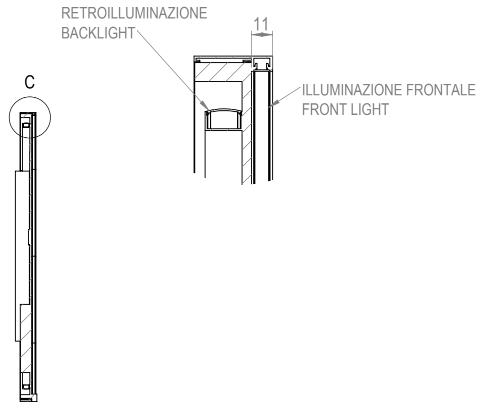
SEZIONE A-A
