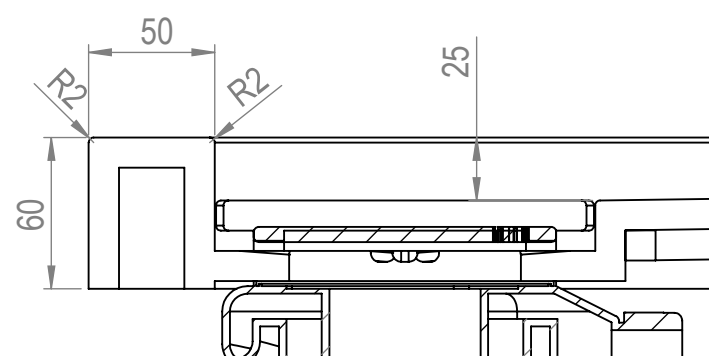
DETTAGLIO H SCALA 1 : 3
