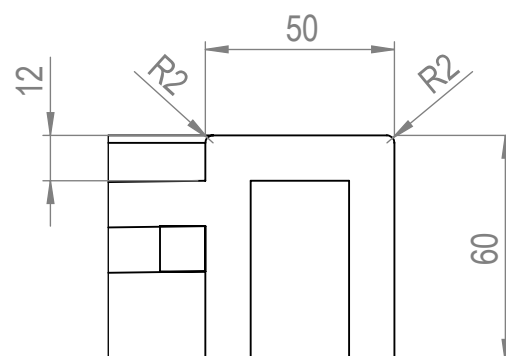
DETTAGLIO G SCALA 1 : 2
