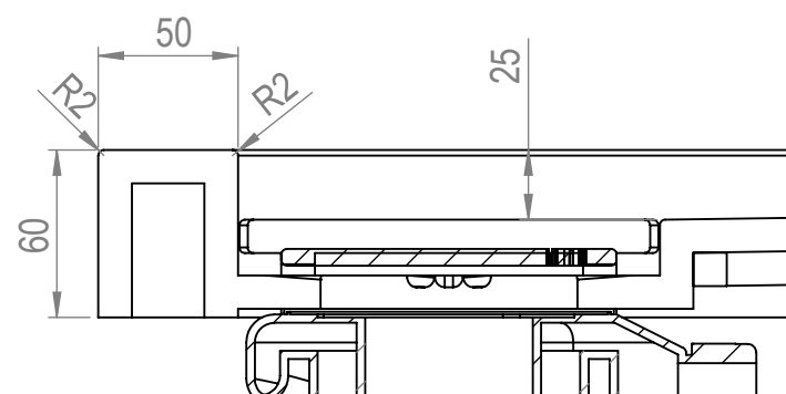
DETTAGLIO D SCALA 1 : 3
