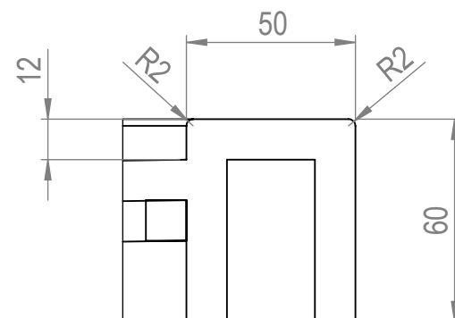
DETTAGLIO C SCALA 1 : 2
