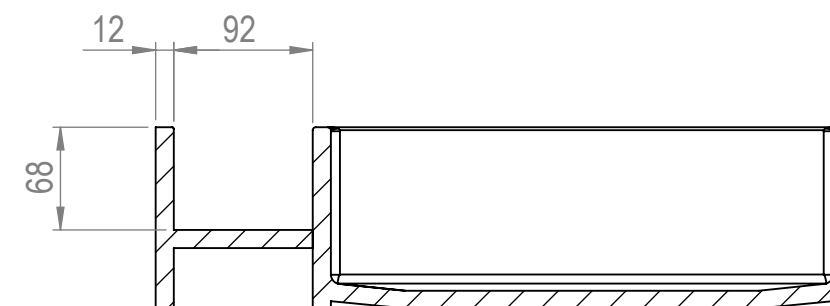
SEZIONE BG-BG
