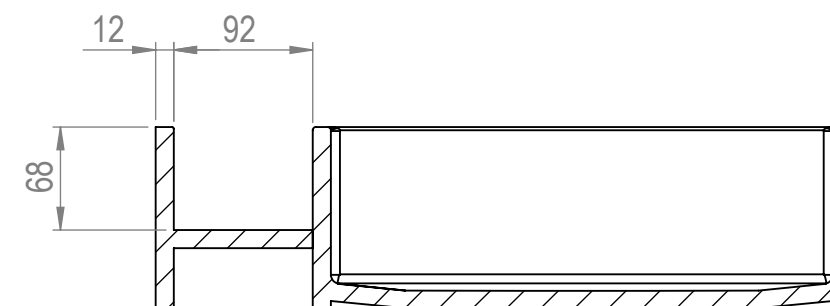
SEZIONE BA-BA
