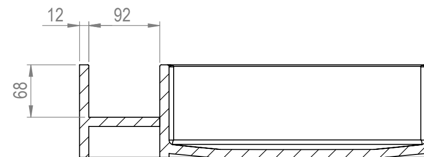
SEZIONE BQ-BQ
