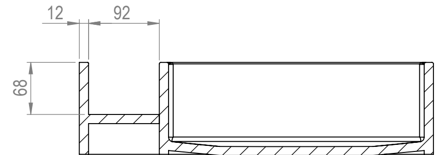
SEZIONE BT-BT
