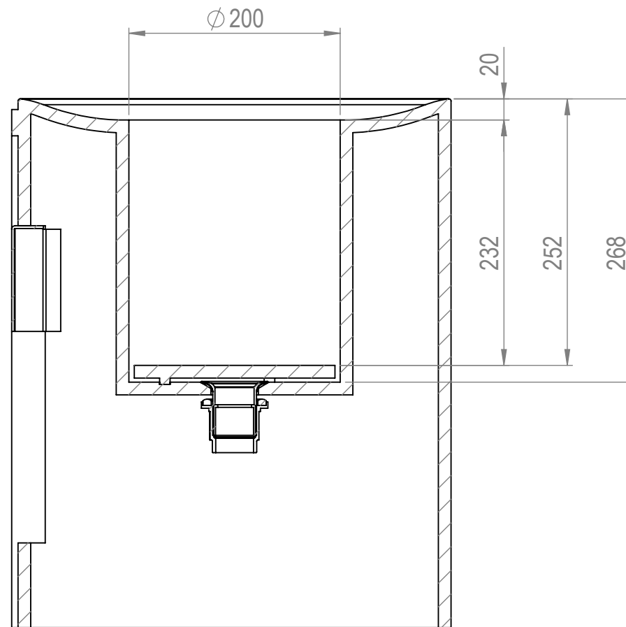
SEZIONE C-C
