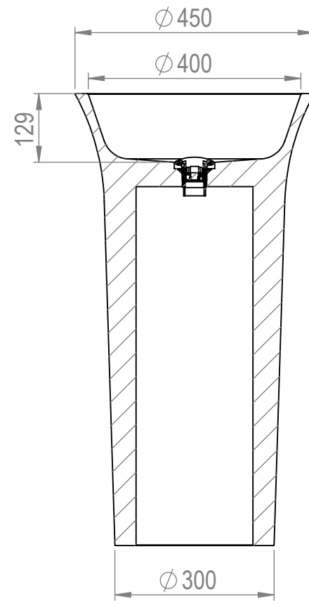
SEZIONE A-A
