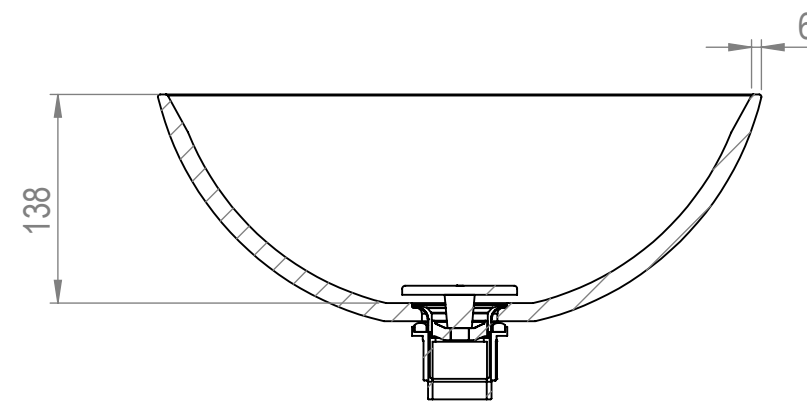
SEZIONE A-A
